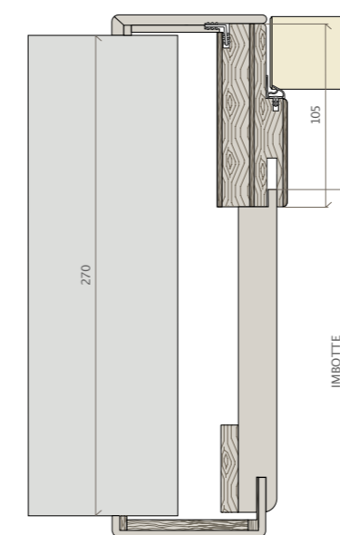
imbotte per spessore muro da 200 a 270 mm compresi jams for wall thickness 200 to 270 cm chambranles pour épaisseur de mur de 200 à 270 cm inclus tapajuntas para paredes de entre 200 y 270 cm de grosor Verblendungen für Wandstärken von 200 bis einschl. 270 cm накладки для стены толщиной от 200 до 270 см включительно
