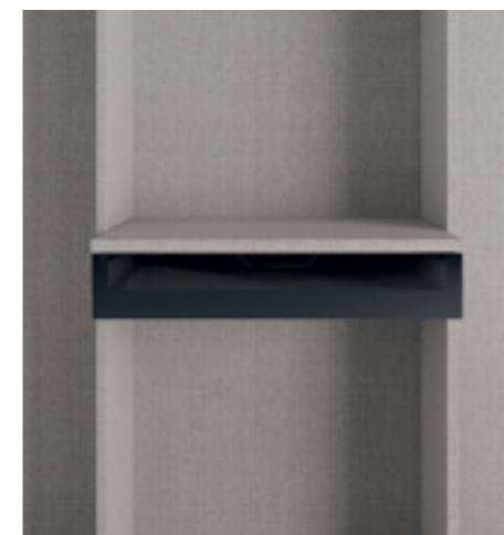
1 cassetto / drawer L 43,7 - 47,7 - 57,3 - 90 - 98 - 117,2 cm
